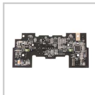
Плата емкостная для купюроприемника CashCode GX
