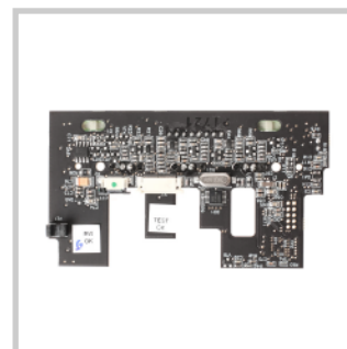
Плата магнитных датчиков для купюроприемника CashCode GX
