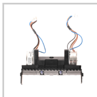
Механизм равнения для купюроприемника CashCode GX
