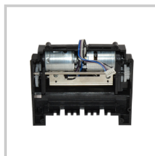
Корпус для купюроприемника CashCode GX
