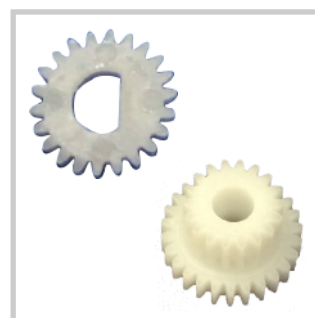
Шестерня [22Т] Шестерня [27Т-18Т]
